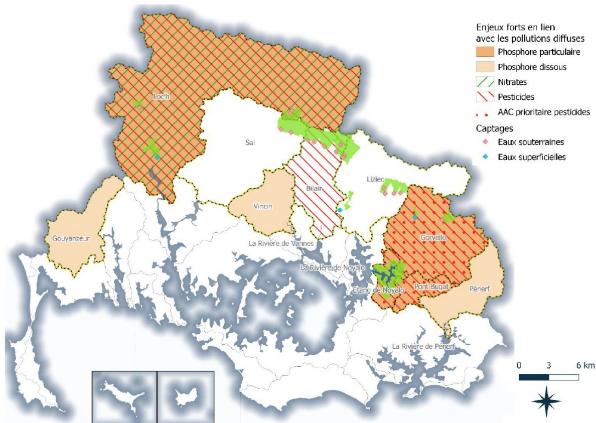
Figure 1: Secteurs prioritaires vis-à-vis de la reconquête de la qualité de l'eau
